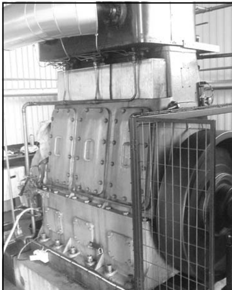
Typ: Cylinderångmaskin Tillverkningsår: 1956 Tillverkare: Bohn und Kähler Varv per minut: 600 rpm Tre st cylindrar, diameter på cylindrarna: 20cm Effekt; ca 30 000 kW/månad
